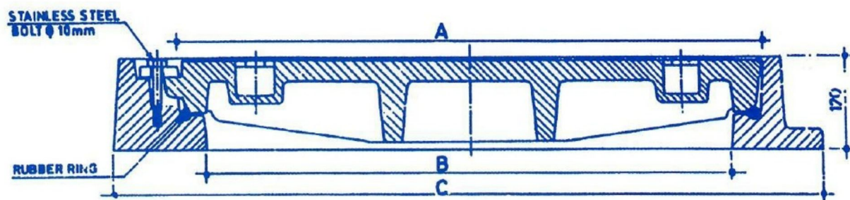
SECTION A-A
